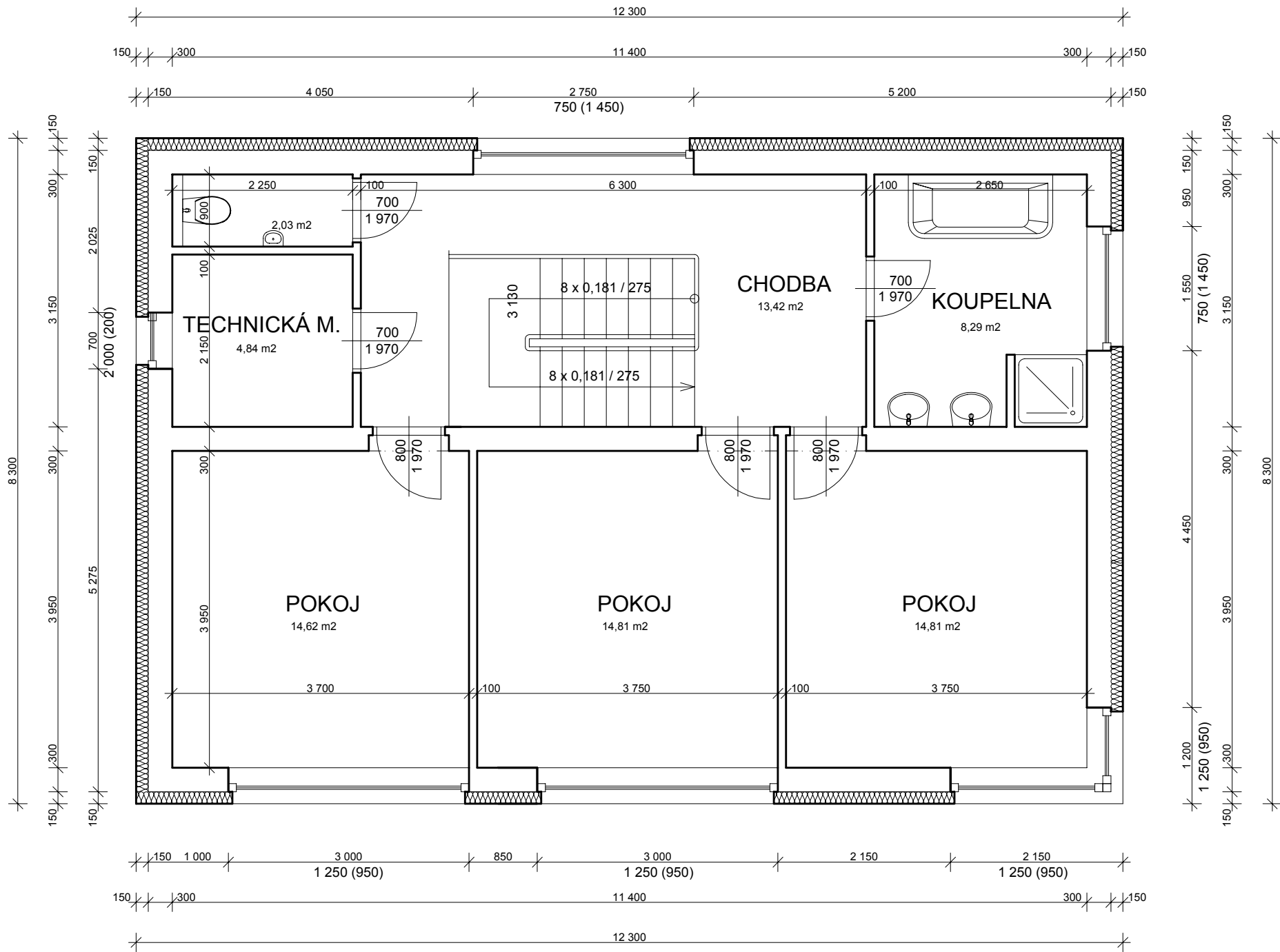
PŮDORYS 2.NP typ B, VAR. ECO
