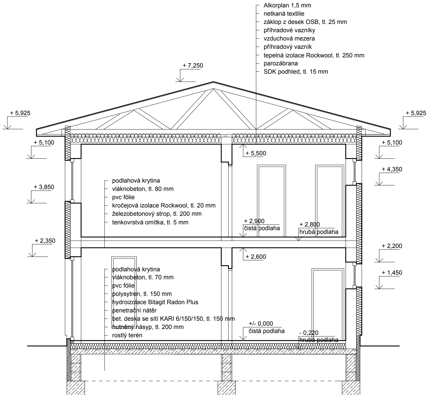
SVISLÝ ŘEZ typ. B, VAR. ECO
