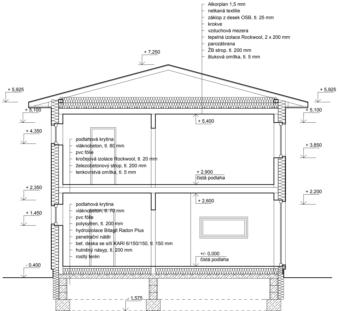
SVISLÝ ŘEZ typ.B, VAR. PASIV
