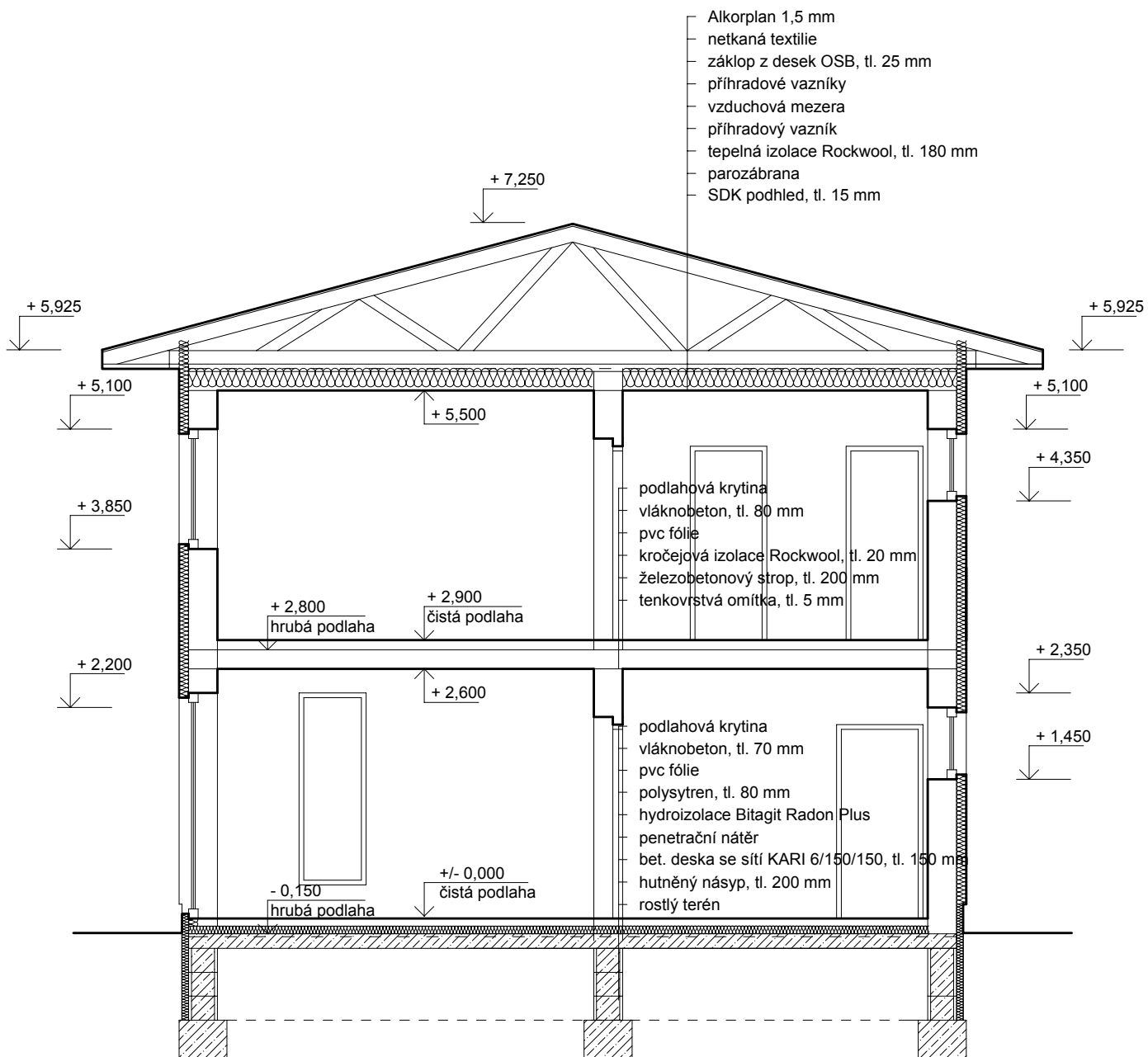
SVISLÝ ŘEZ typ. B, VAR. STANDARD
