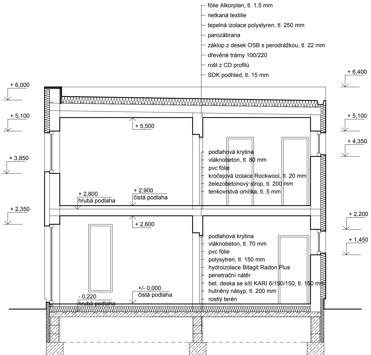
SVISLÝ ŘEZ typ. B, VAR. ECO
