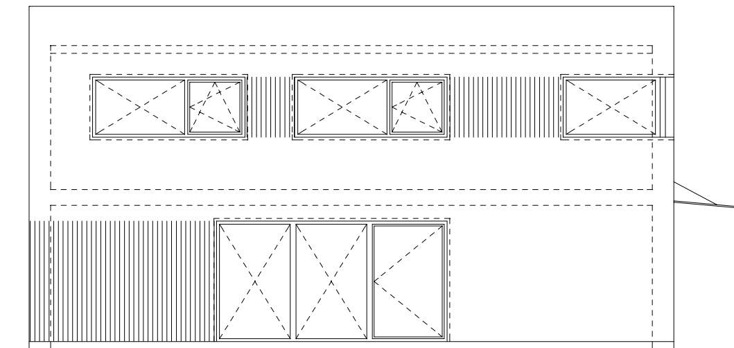
POHLED Z JIHU
