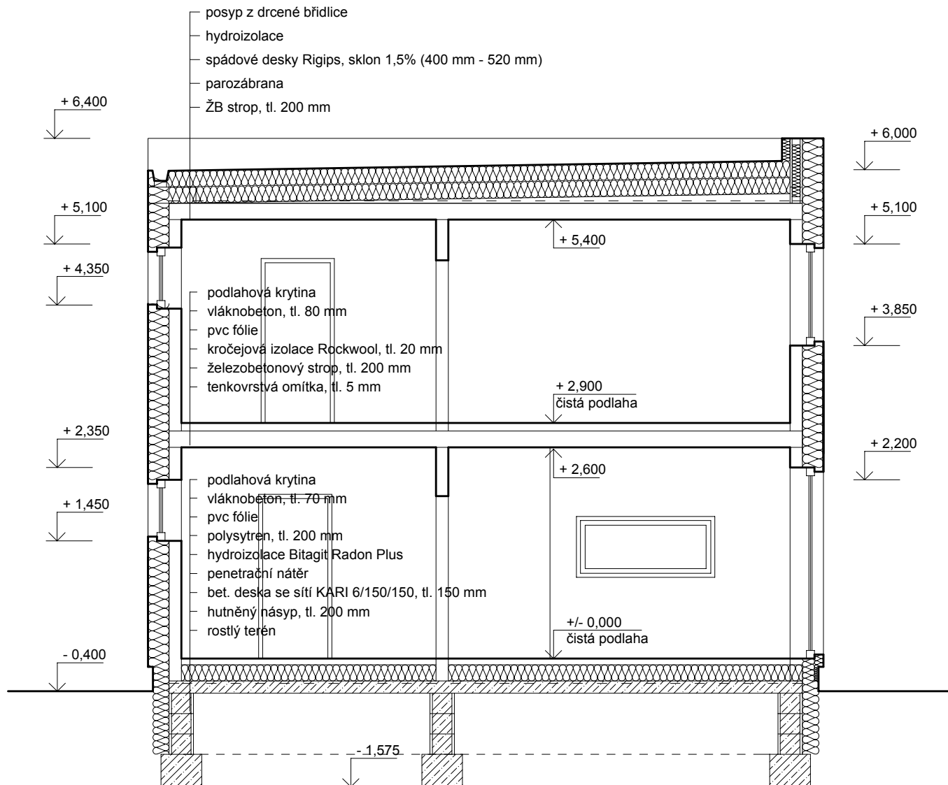
SVISLÝ ŘEZ typ. B, VAR. PASIV
