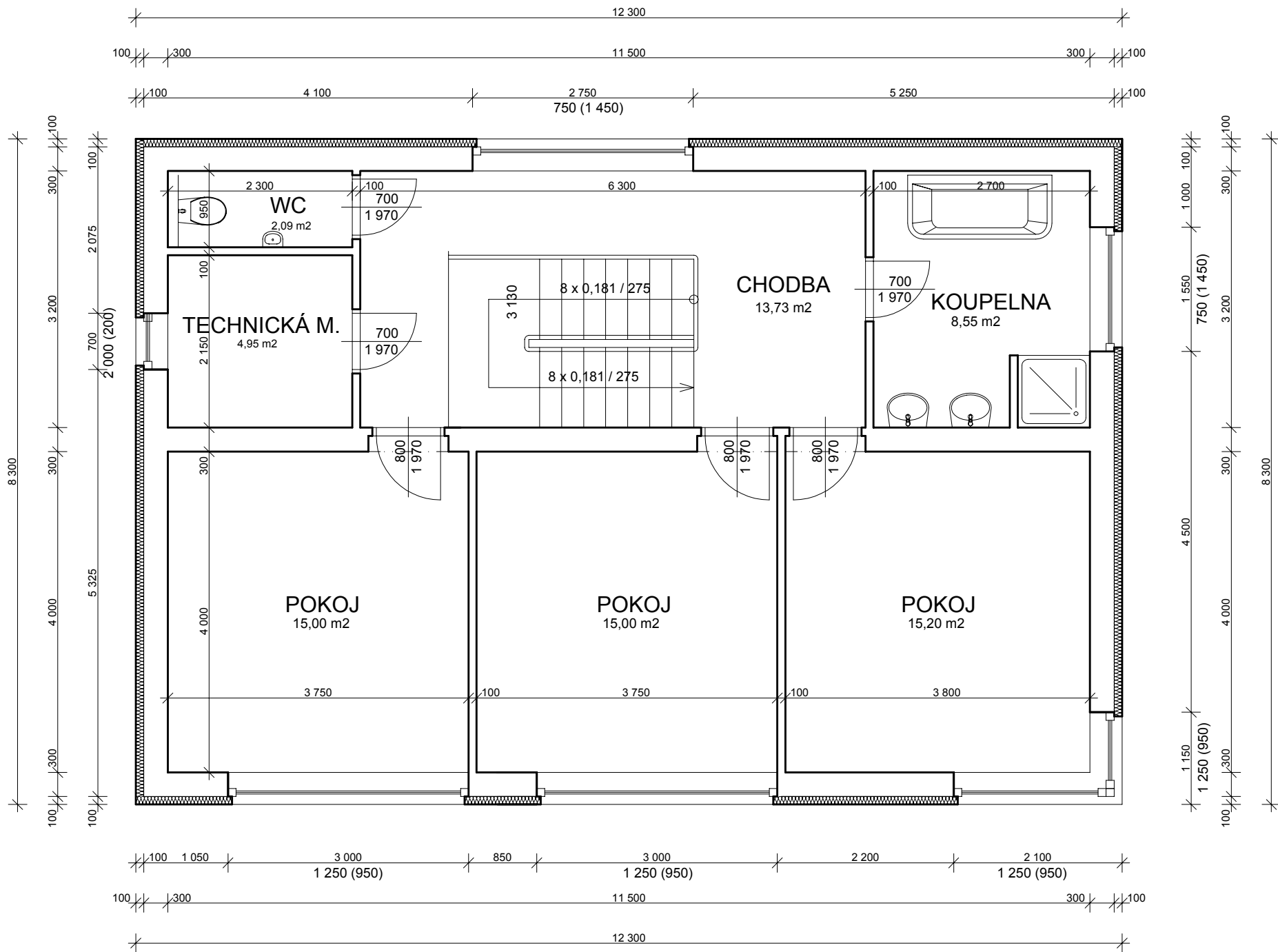
PŮDORYS 2.NP typ B, VAR. STANDARD
