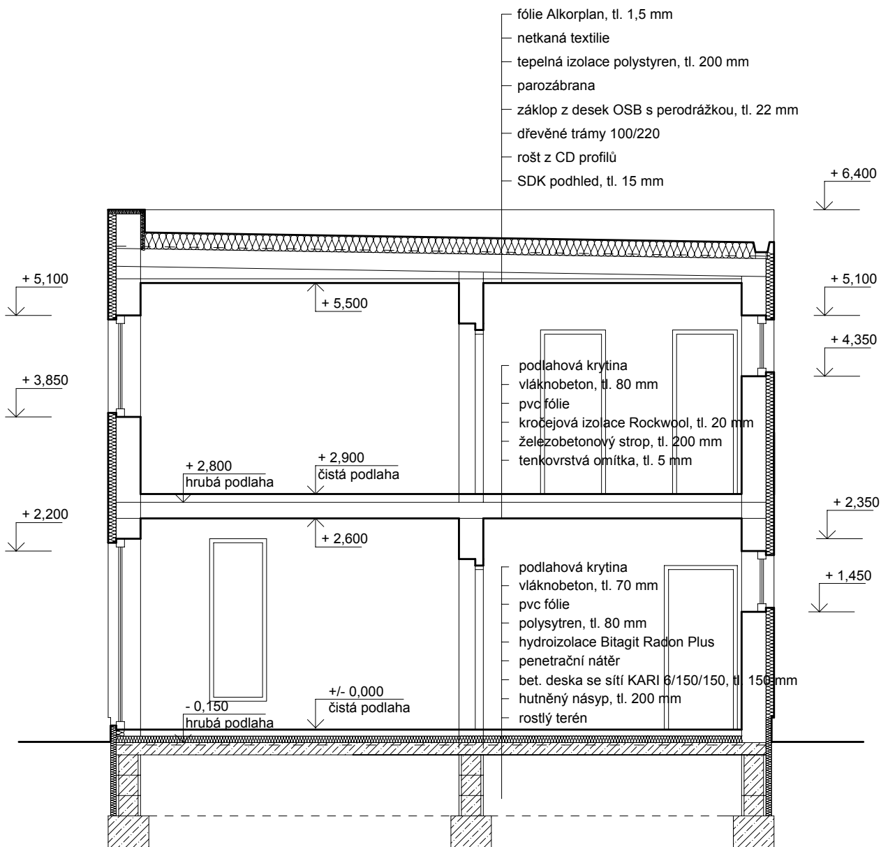
SVISLÝ ŘEZ typ. B, VAR. STANDARD
