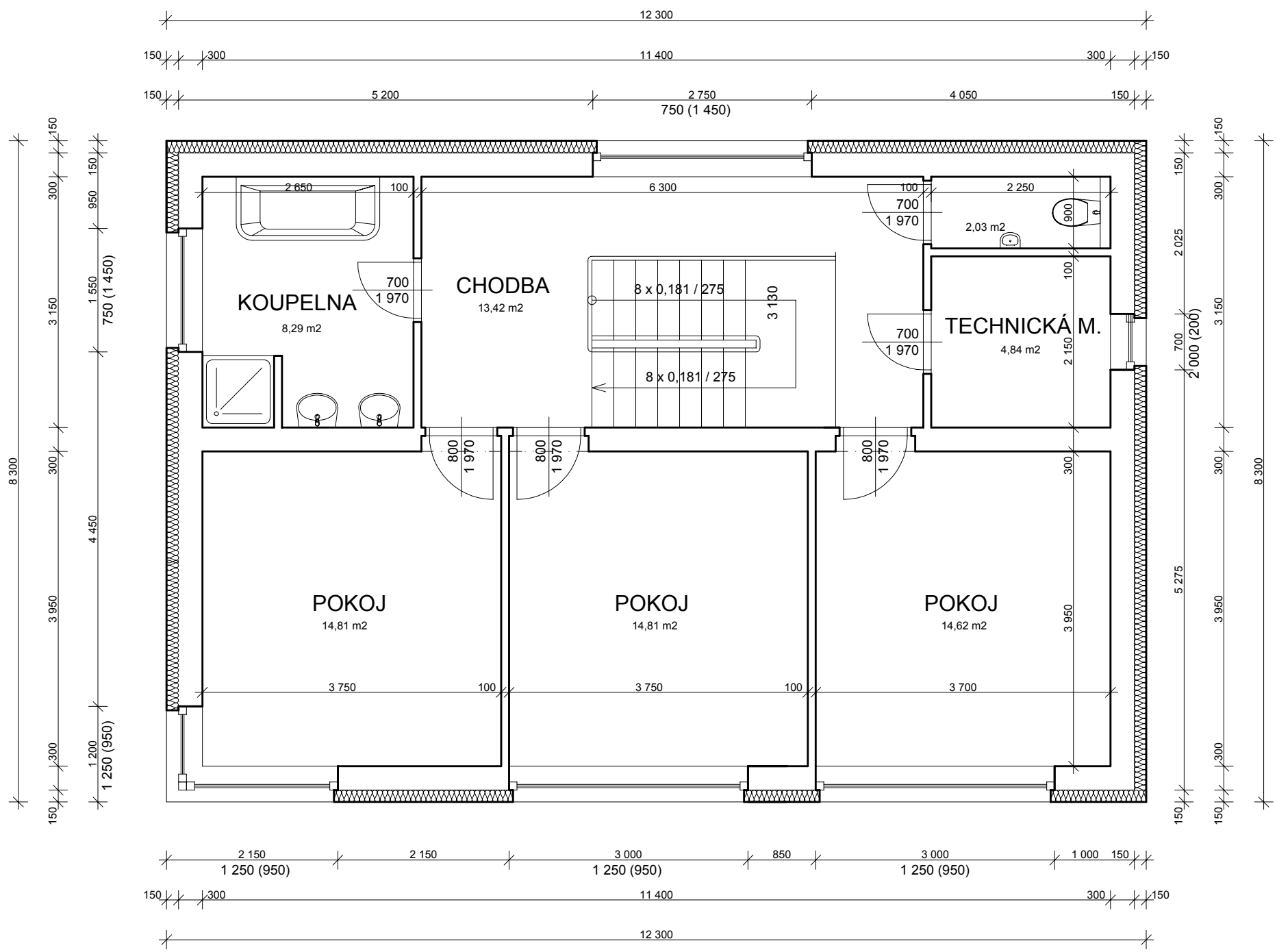
PŮDORYS 2.NP typ A, VAR. ECO
