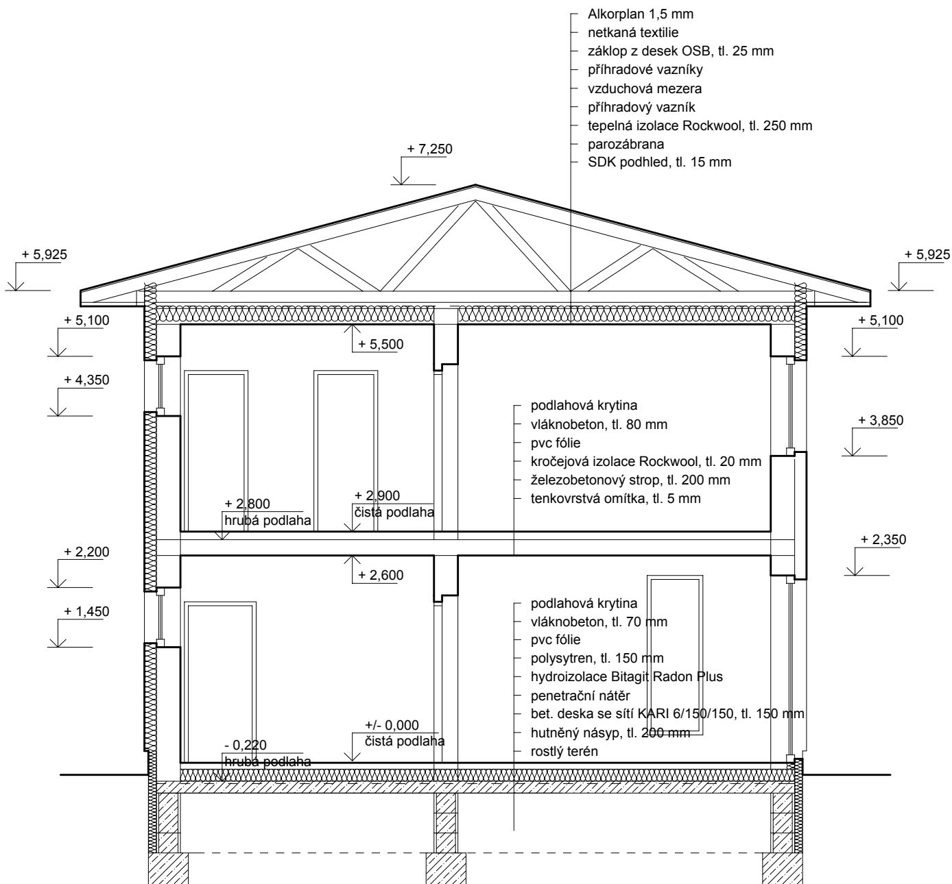
SVISLÝ ŘEZ typ. A, VAR. ECO
