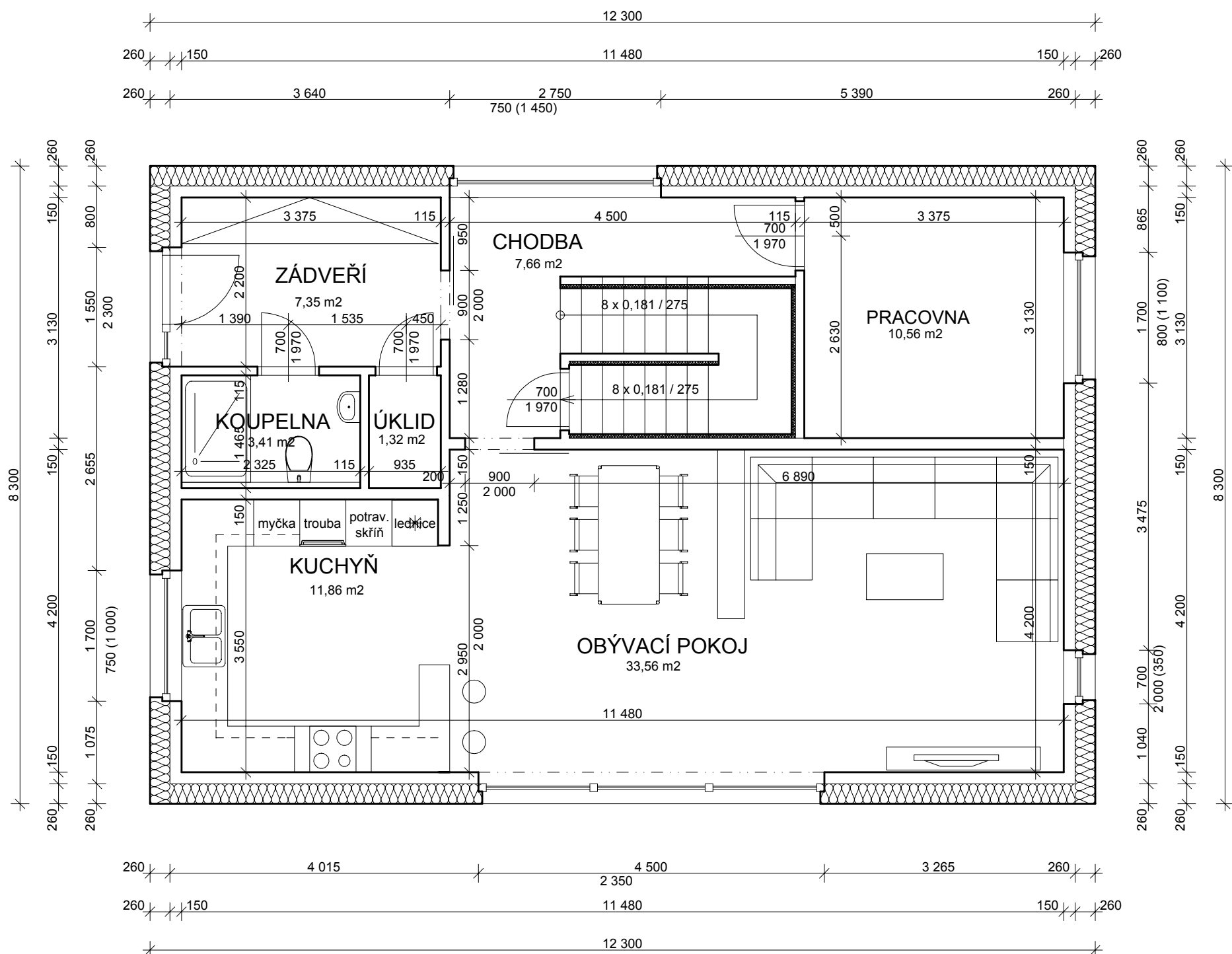
PŮDORYS 1.NP typ. A, VAR. PASIV
