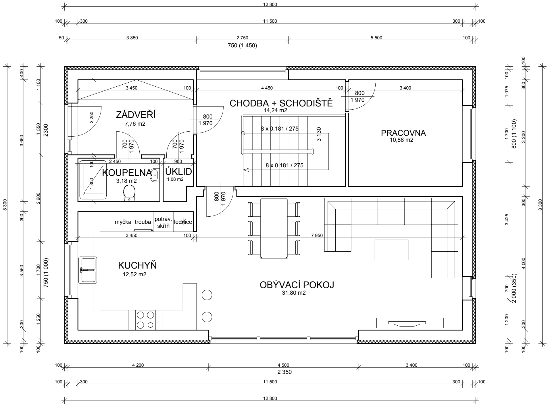
PŮDORYS 1.NP typ. A, VAR. STANDARD
