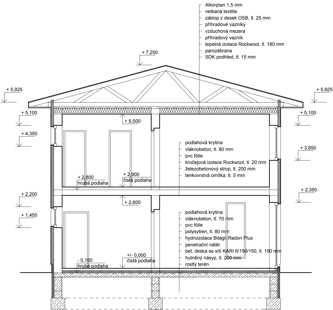
SVISLÝ ŘEZ typ. A, VAR. STANDARD
