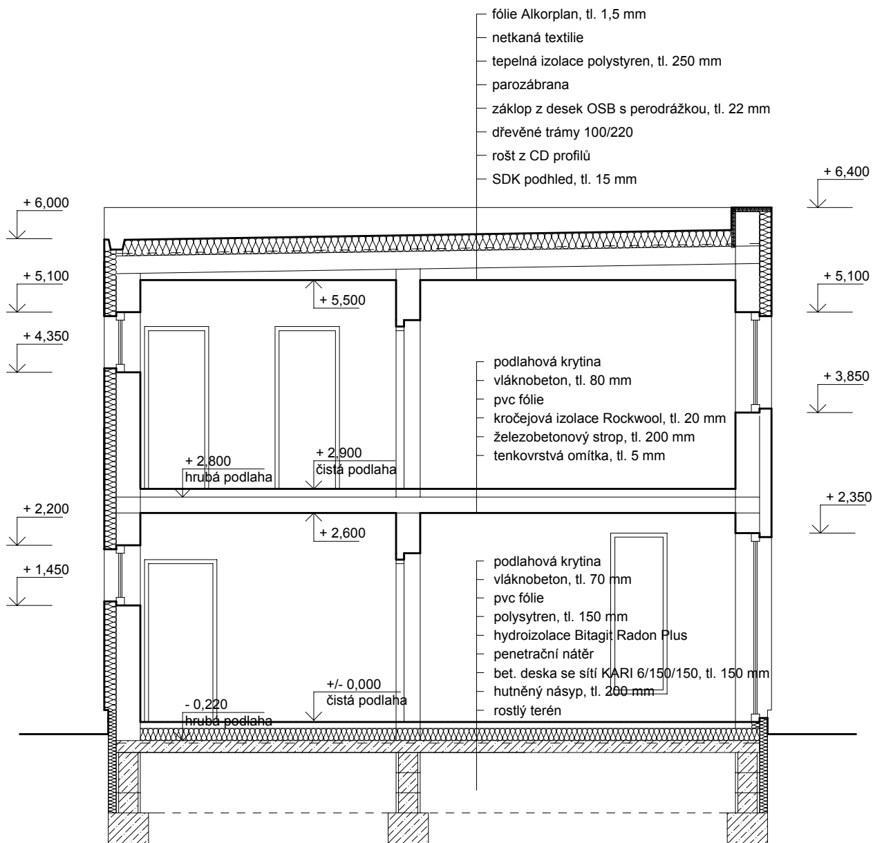
SVISLÝ ŘEZ typ. A, VAR. ECO
