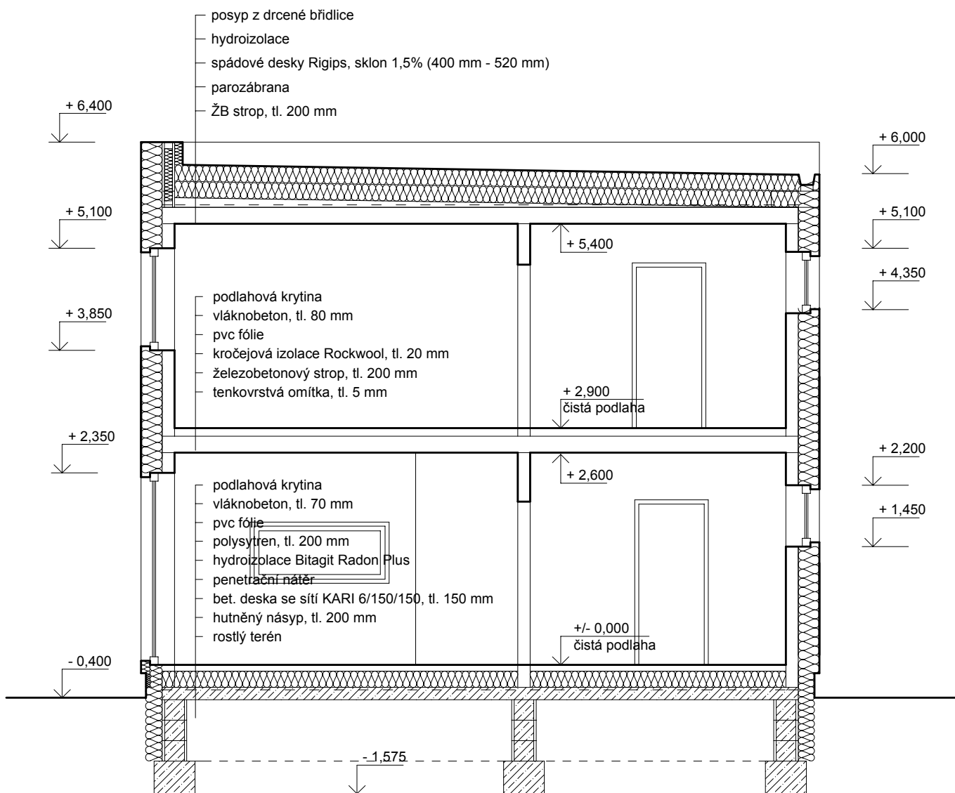
SVISLÝ ŘEZ typ. A, VAR. PASIV
