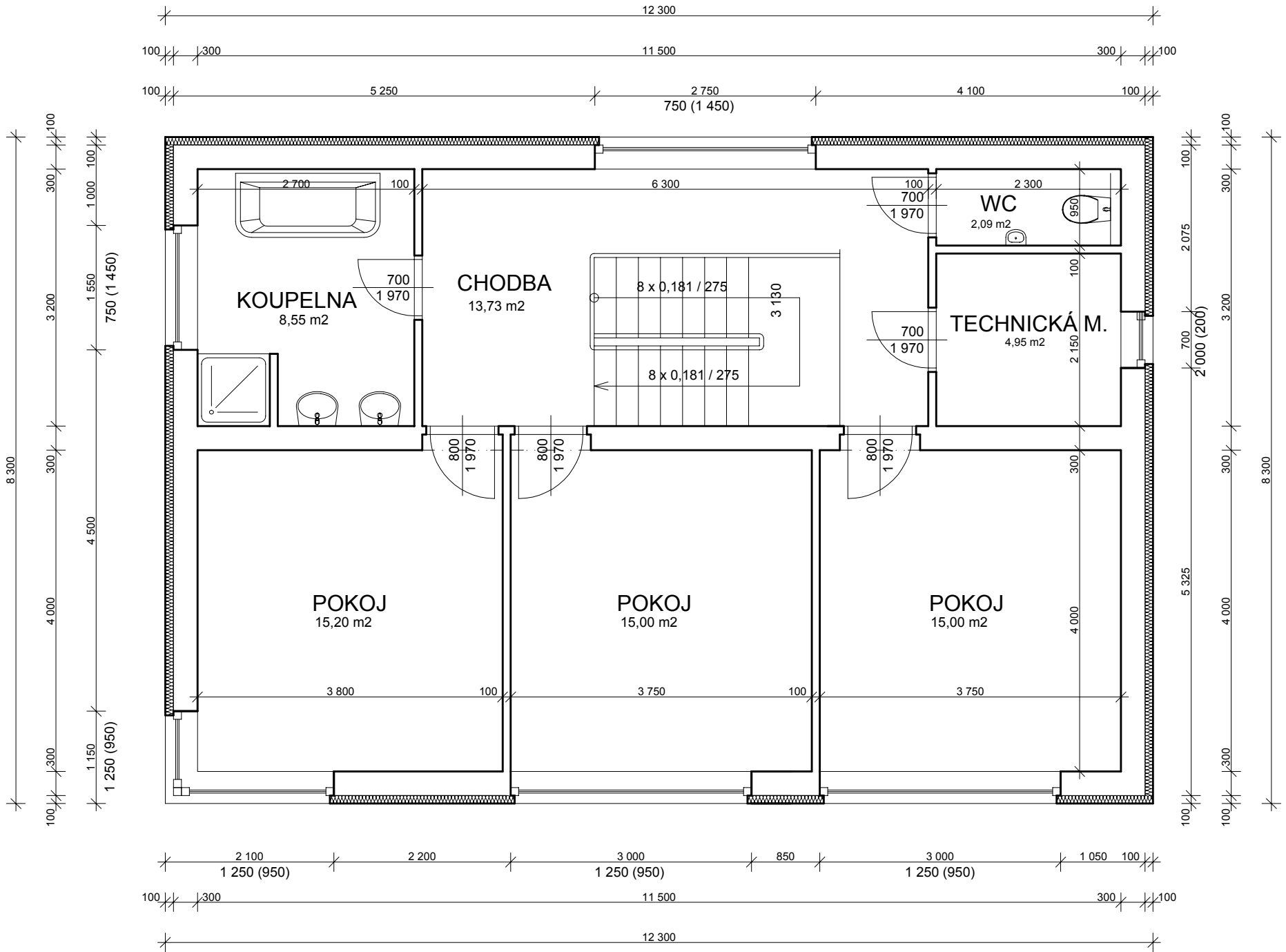
PŮDORYS 2.NP typ A, VAR. STANDARD
